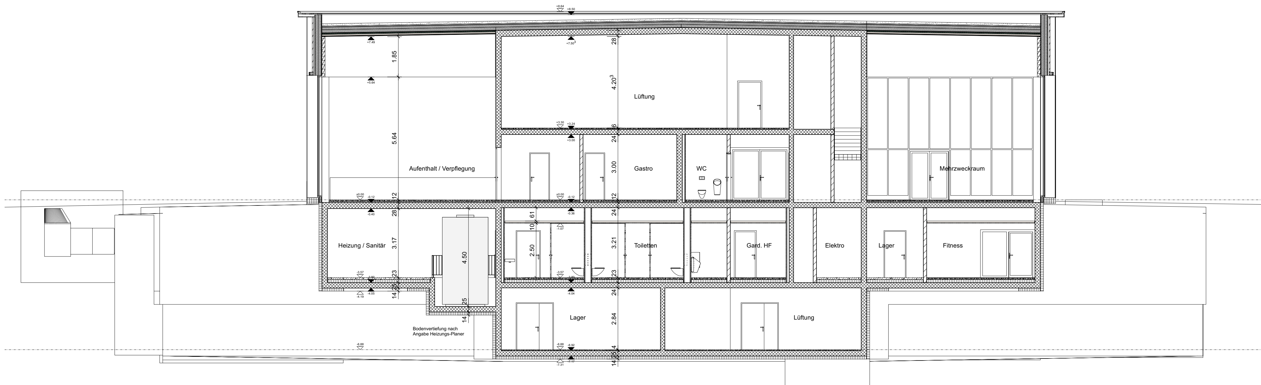
Querschnitt Y-Y (Kern)
